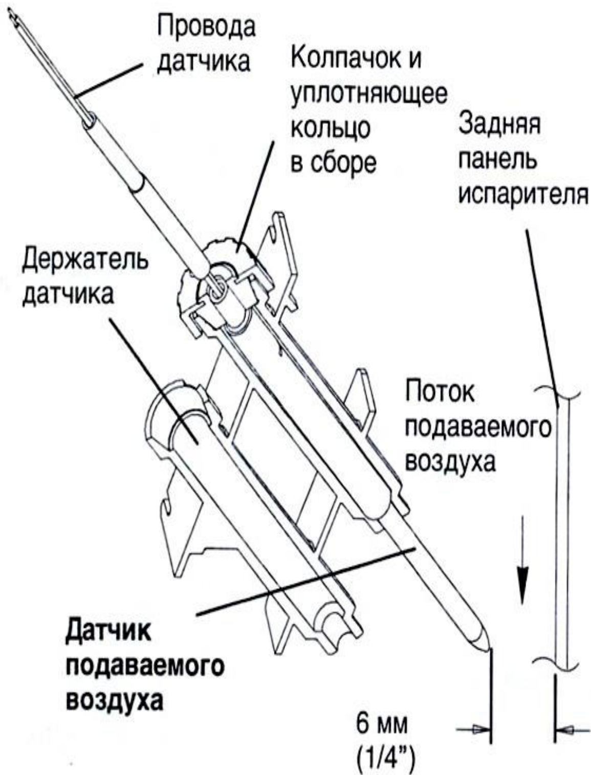
Рис.6-22. Положение датчика подаваемого воздуха
