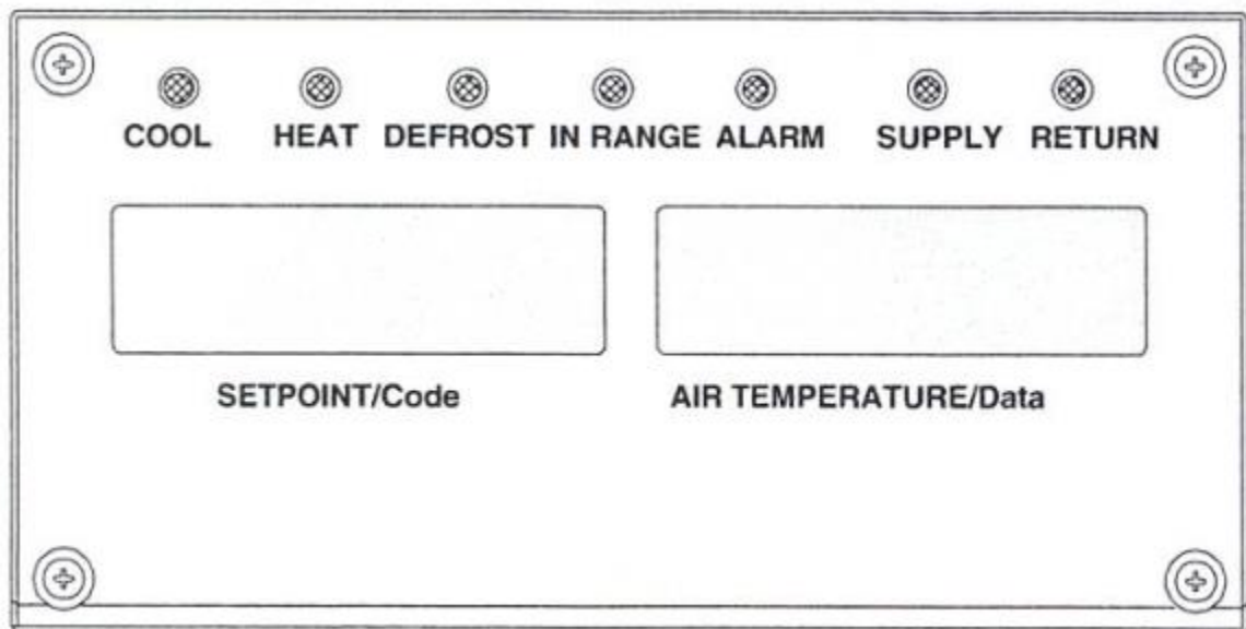
Рис. 3-3. Блок дисплея
