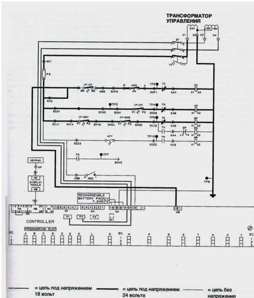
Рис. 4-1 Режим охлаждения
