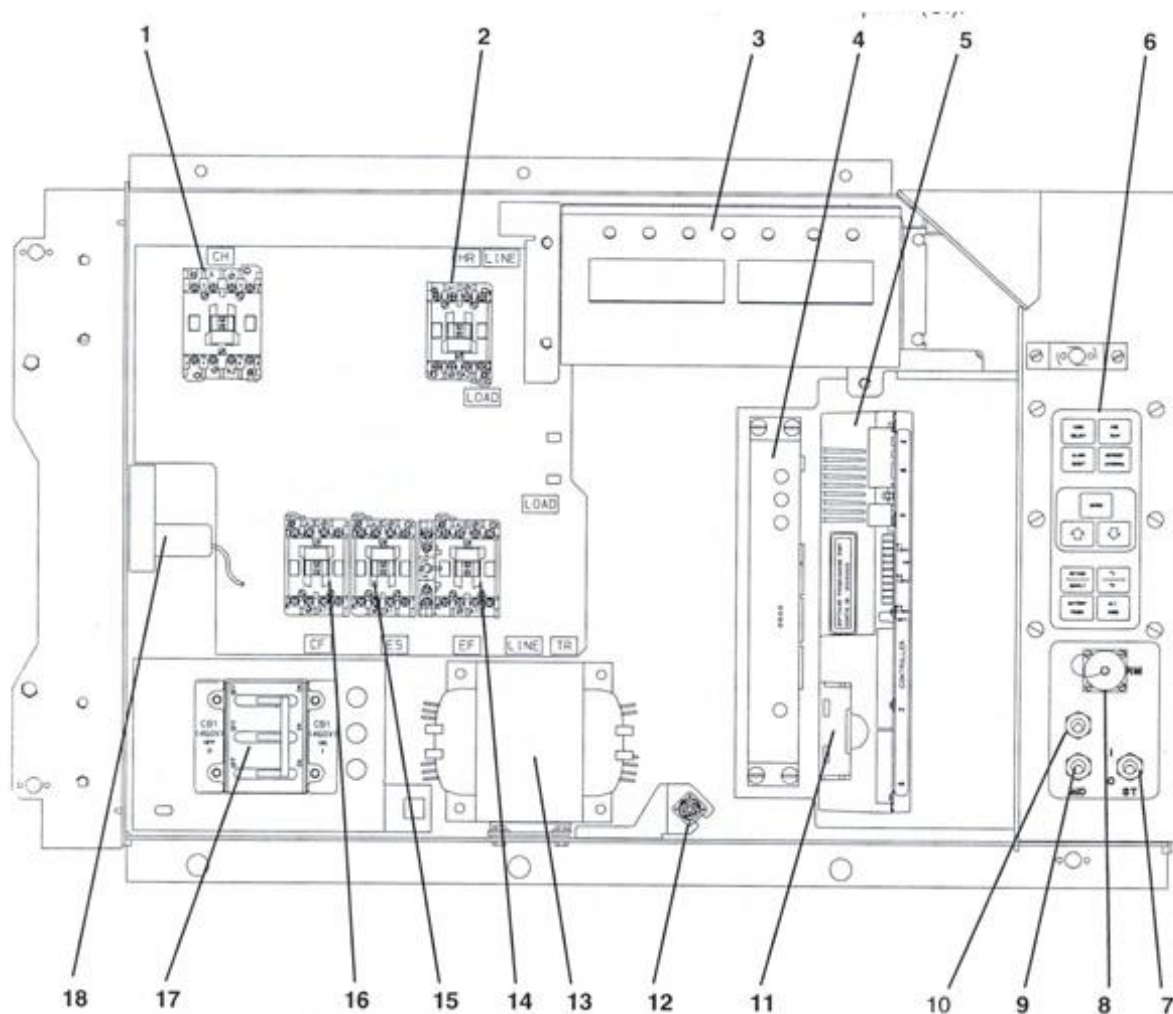
Рис. 2-7. Отсек управления
