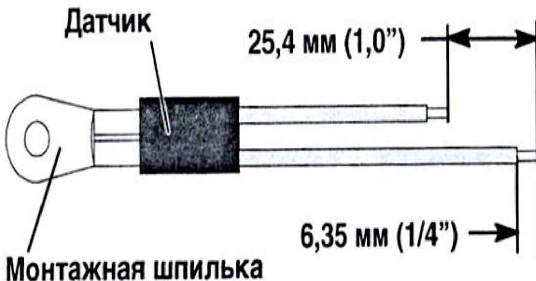
Рис. 6-26. Датчик (AMBS или DTS)
