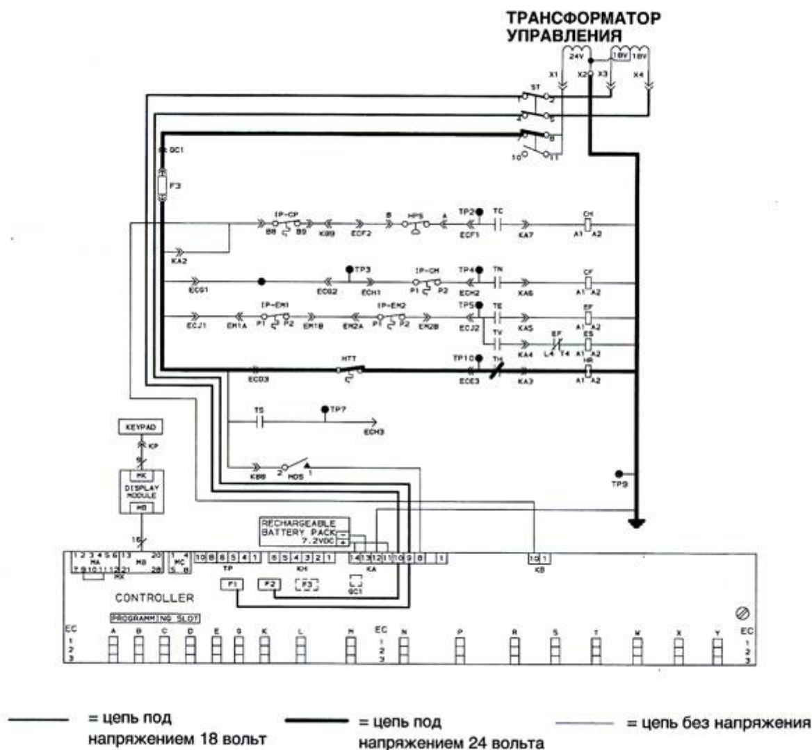
Рис. 4-3. Режим оттаивания
