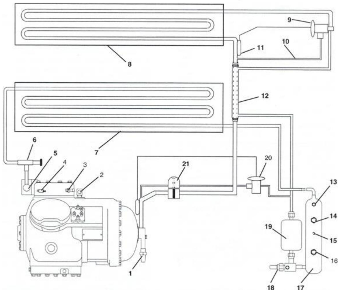
Рис. 2-9. Холодильный контур со сборником хладогена
