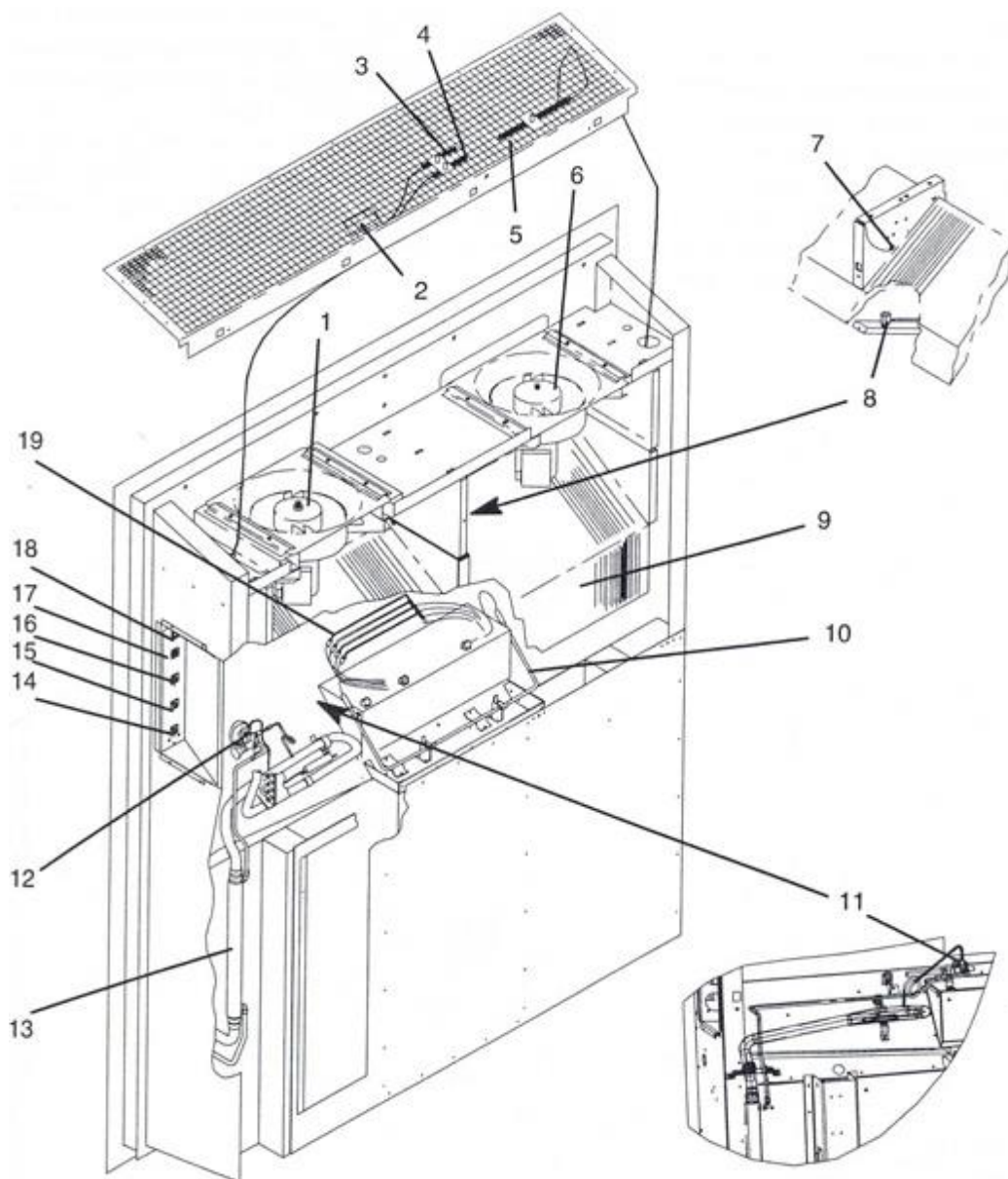
Рис. 2-2. Отсек испарителя
