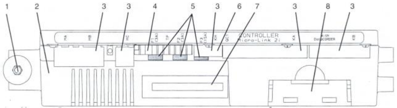
Рис. 3-1. Блок контроллера/ DataCORDER Micro-Link 2i
