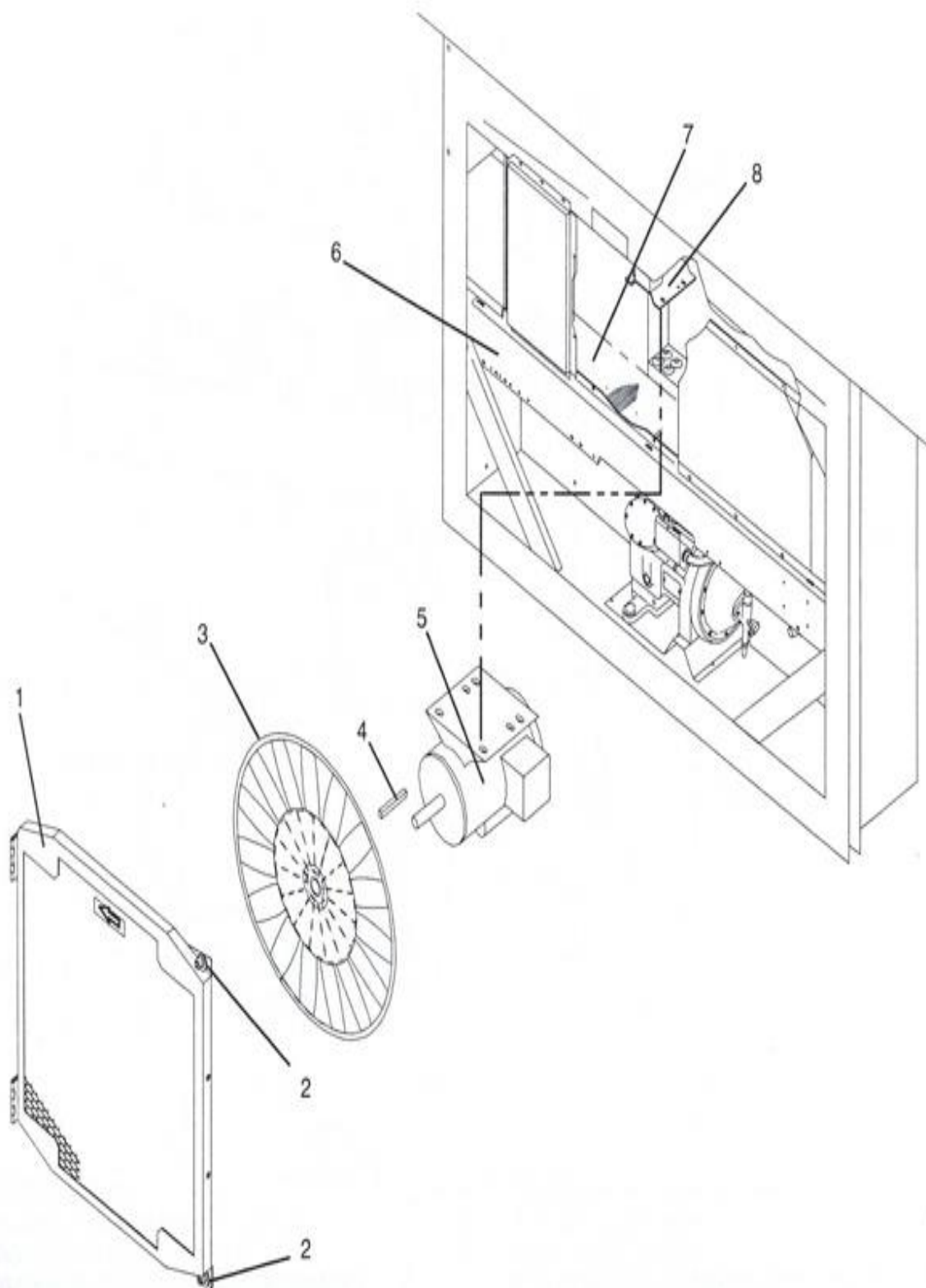
Рис. 2-4. Отсек конденсатора
