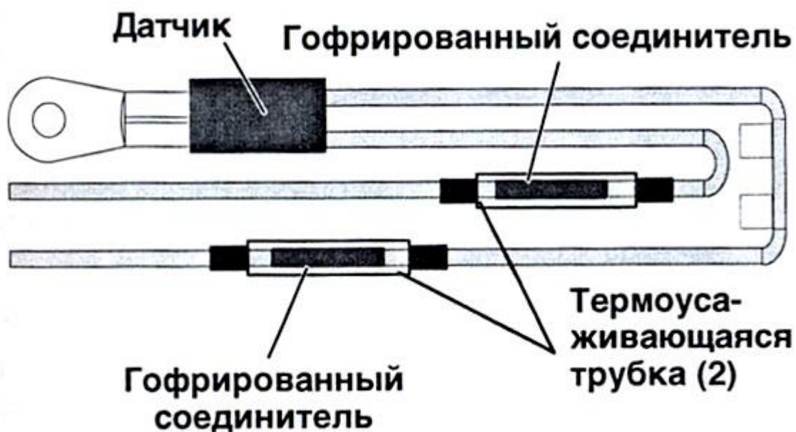
Рис.6-27. Датчик в сборе с проводами (AMBS или DTS)
