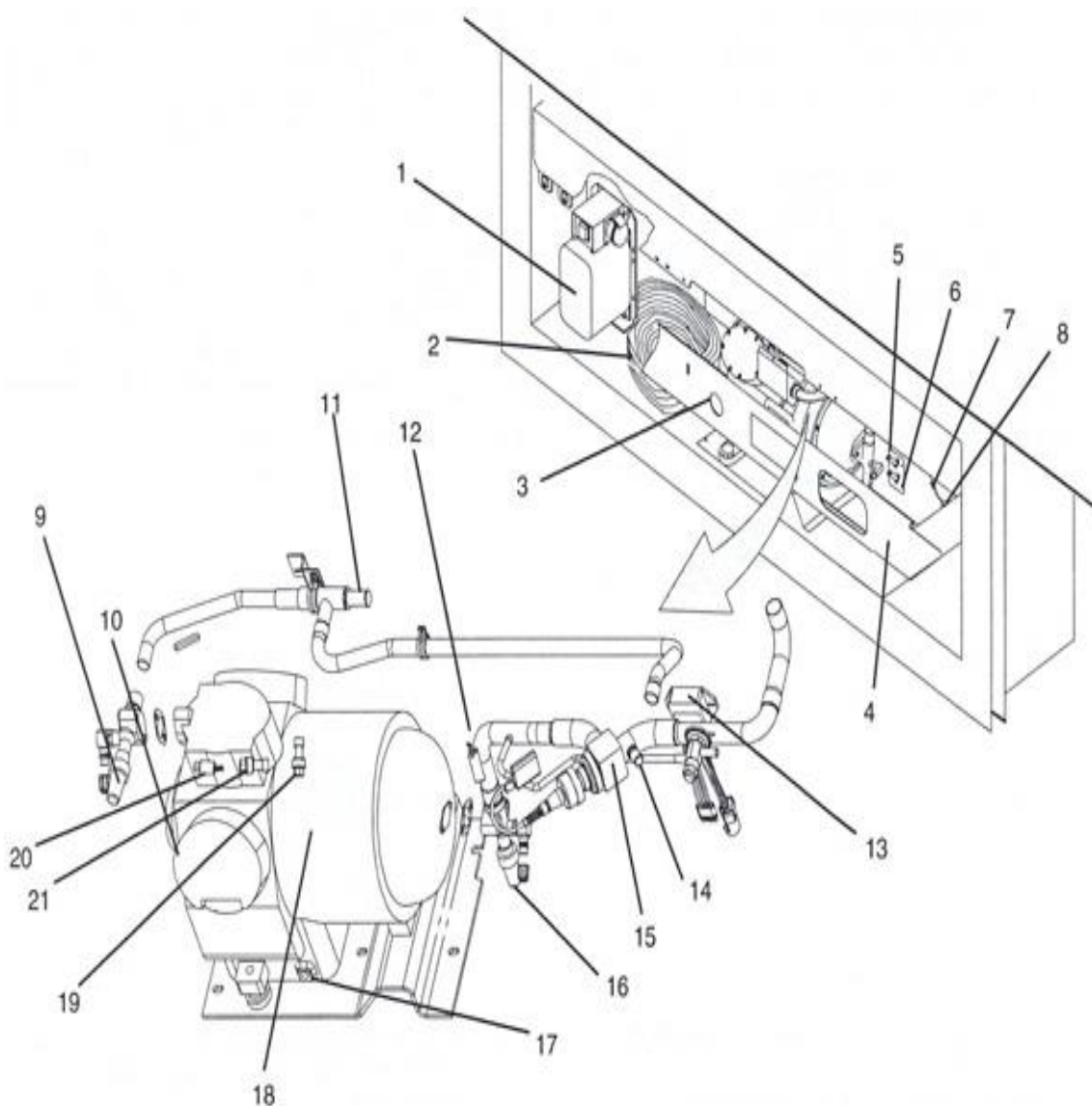
Рис. 2-3. Отсек компрессора
