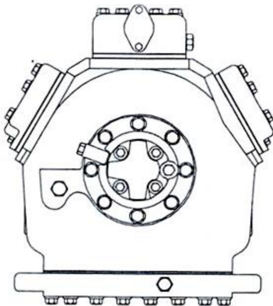
Рис.6-16. Маслонасос компрессора; вид с торца
